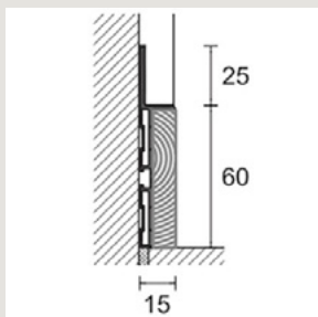
Grindjuostė, įleidžiama į sieną 60 x 2000 x 15mm
